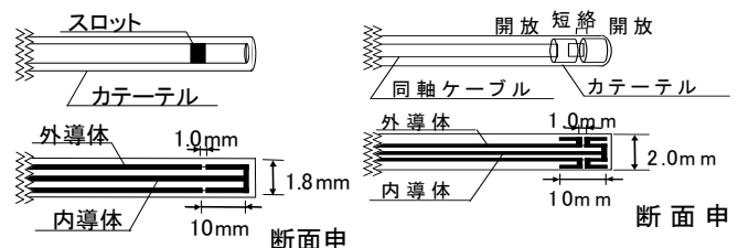
図 2 アンテナの構造
